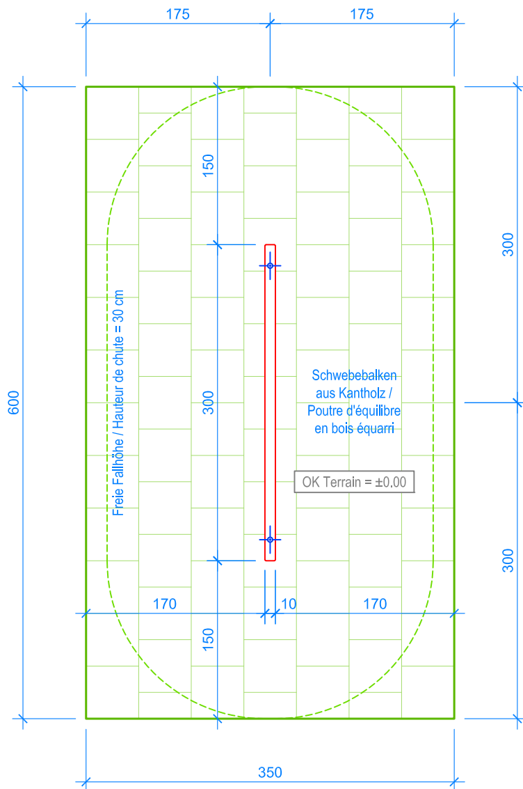
GRUNDRISS / PLAN 1:50
