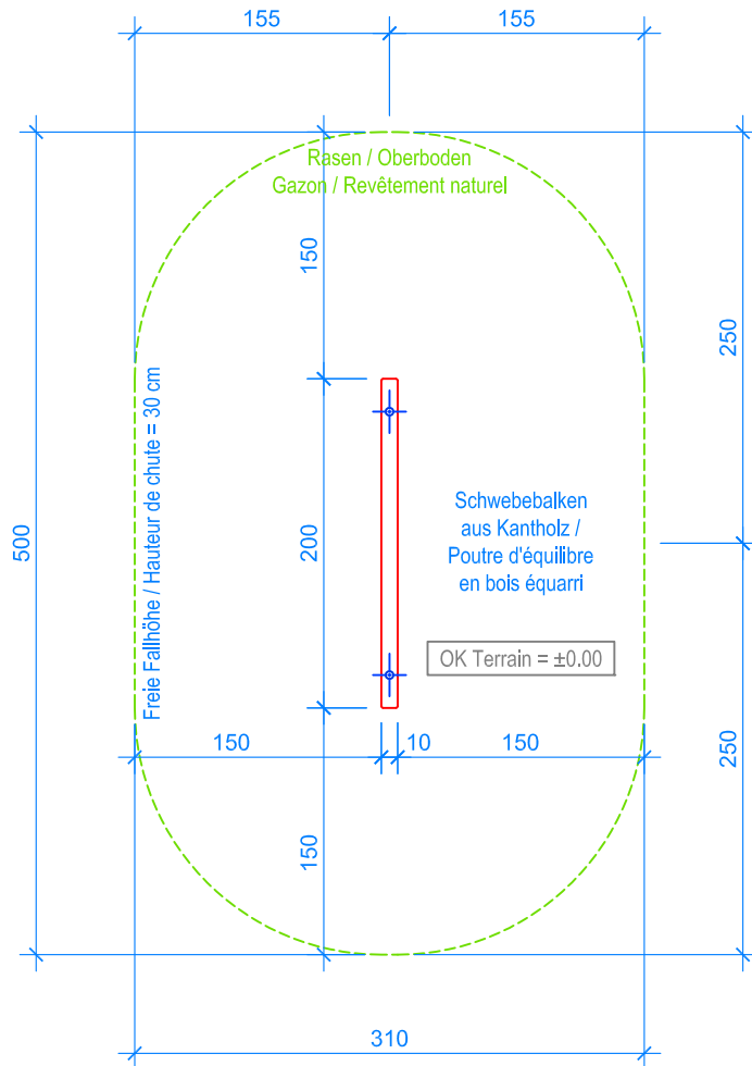
GRUNDRISS / PLAN 1:50
