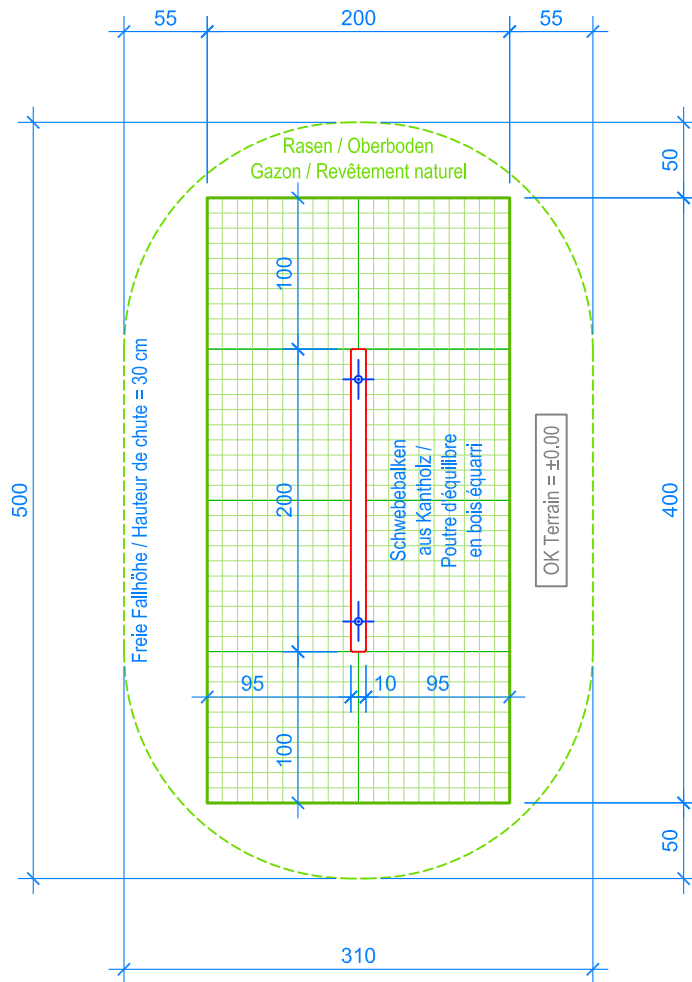
GRUNDRISS / PLAN 1:50
