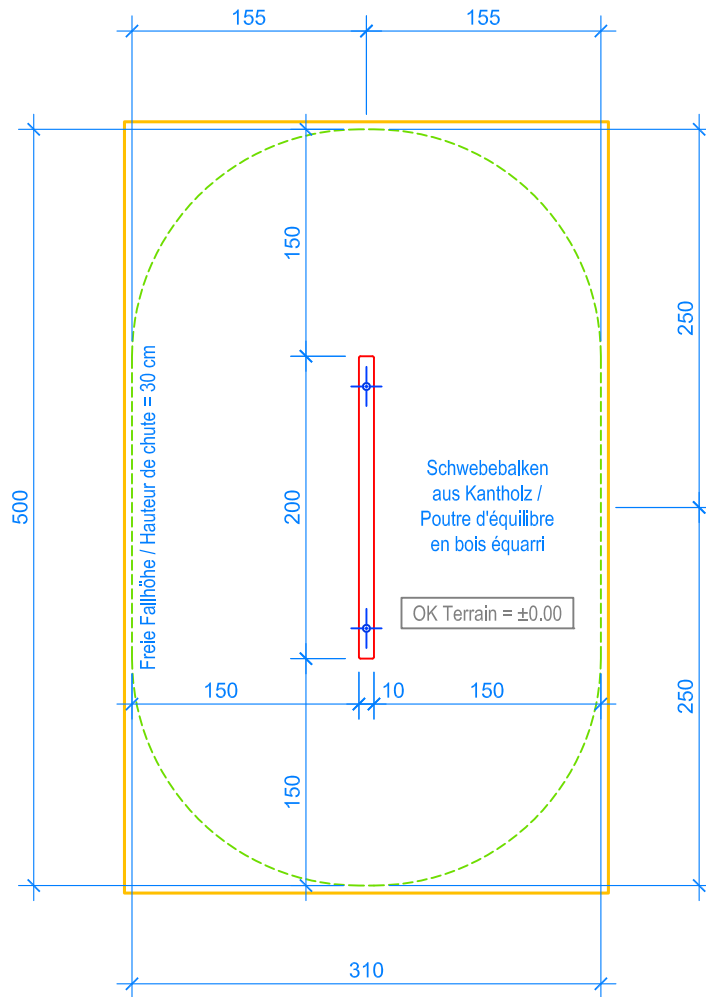
GRUNDRISS / PLAN 1:50
