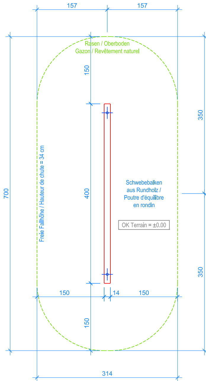
GRUNDRISS / PLAN 1:50
