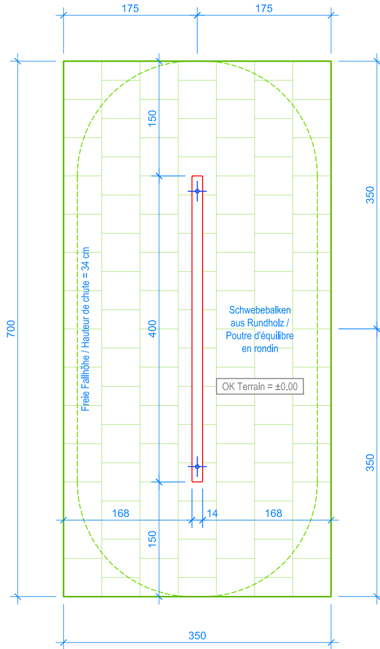
GRUNDRISS / PLAN 1:50
