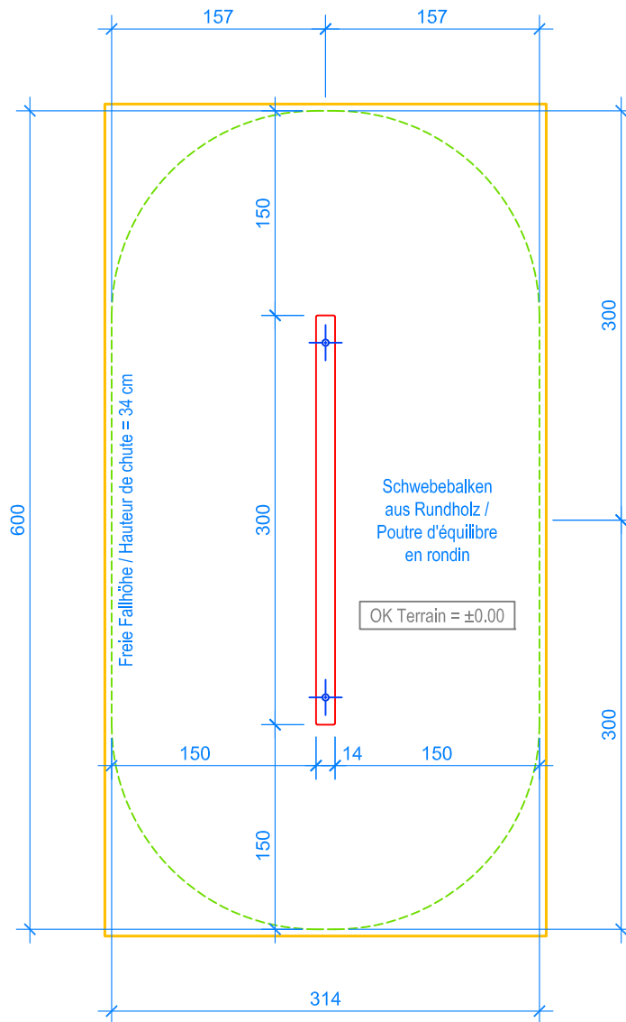
GRUNDRISS / PLAN 1:50
