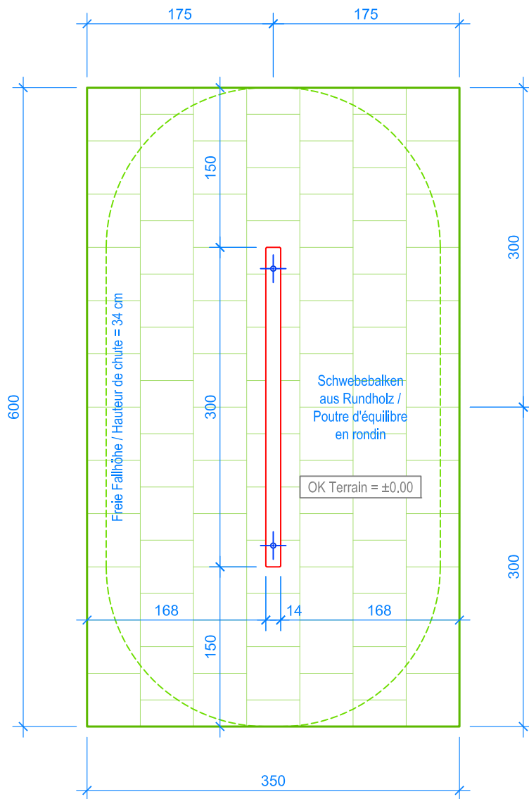
GRUNDRISS / PLAN 1:50
