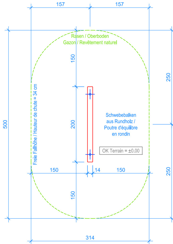
GRUNDRISS / PLAN 1:50
