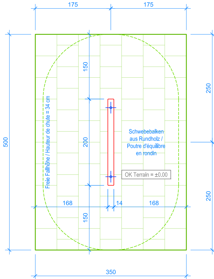
GRUNDRISS / PLAN 1:50
