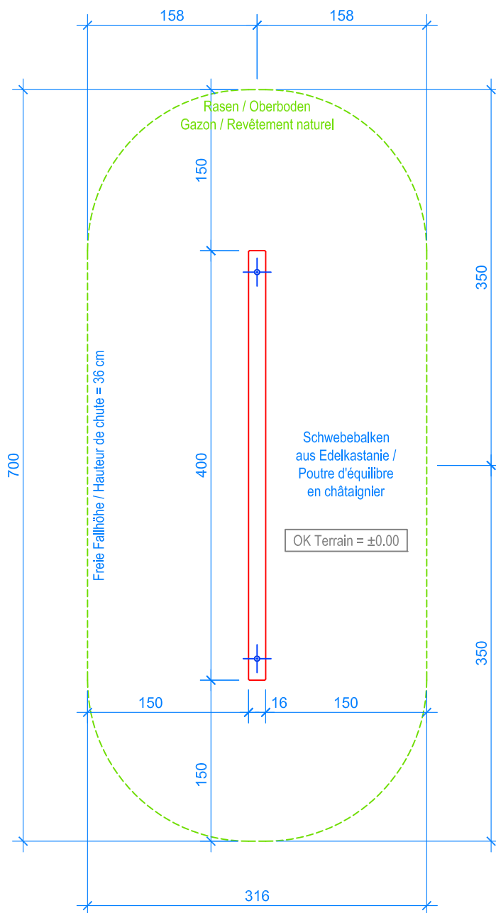
GRUNDRISS / PLAN 1:50
