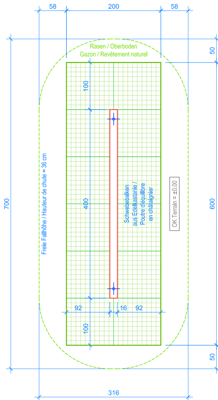
GRUNDRISS / PLAN 1:50
