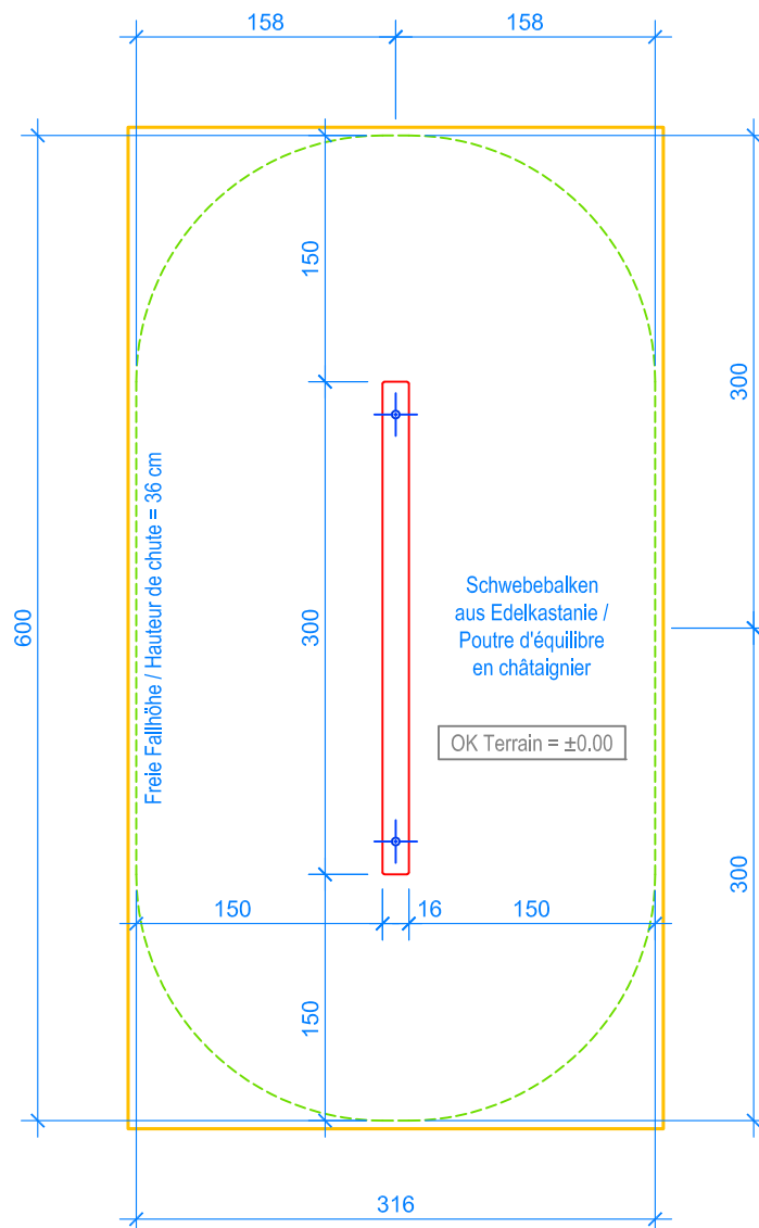
GRUNDRISS / PLAN 1:50
