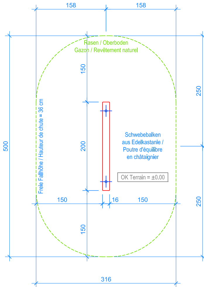
GRUNDRISS / PLAN 1:50
