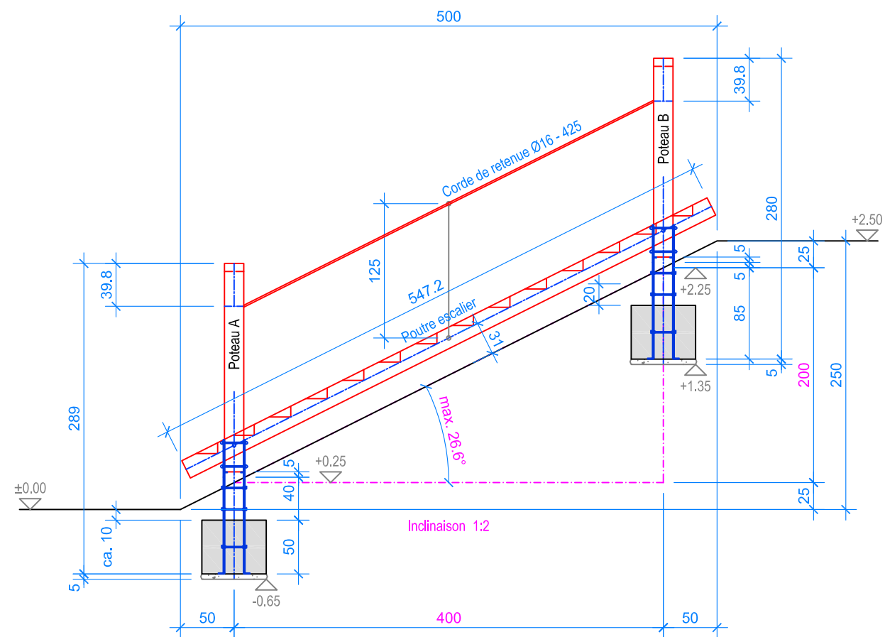
COUPÉ 1:50
