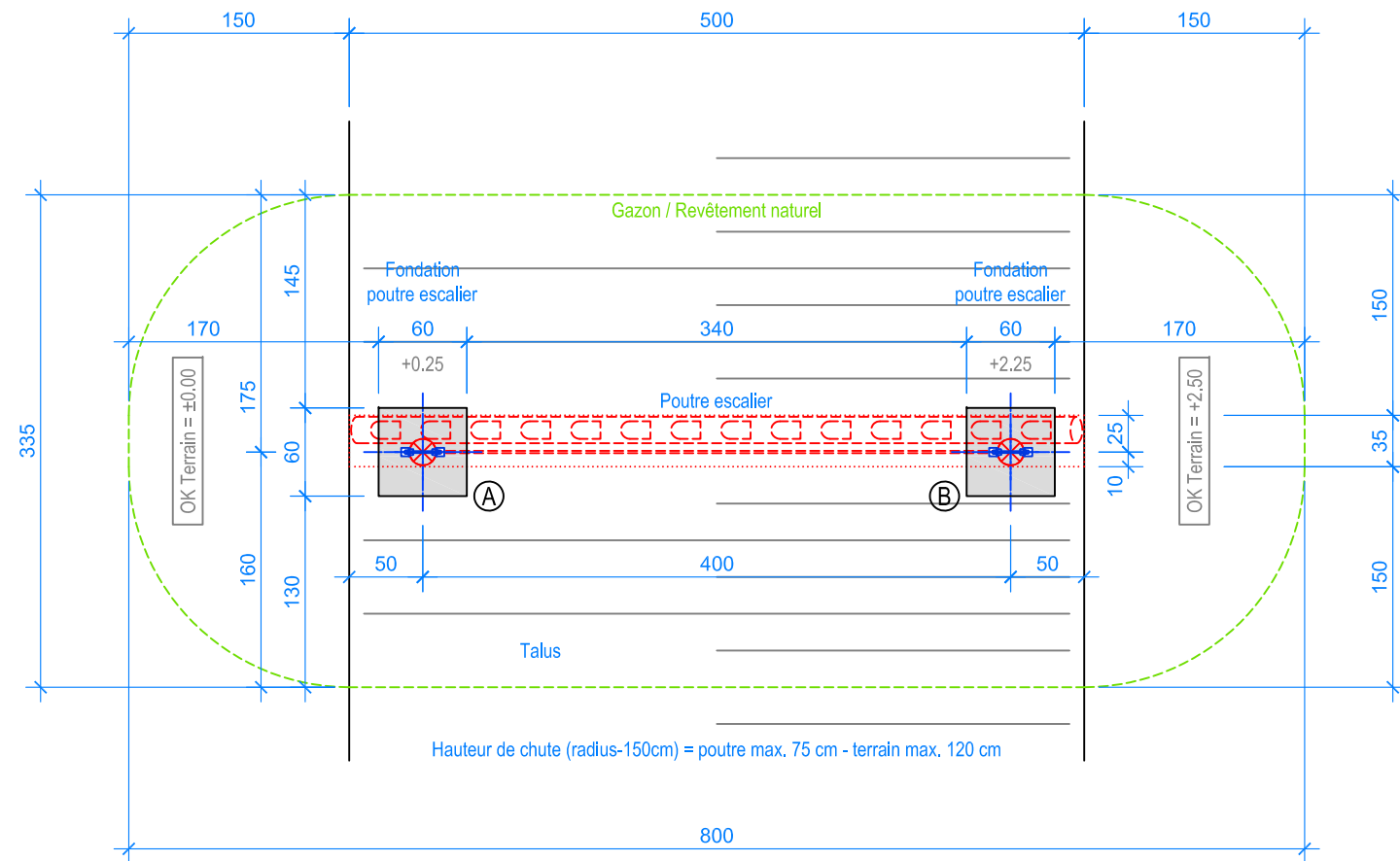
PLAN 1:50
