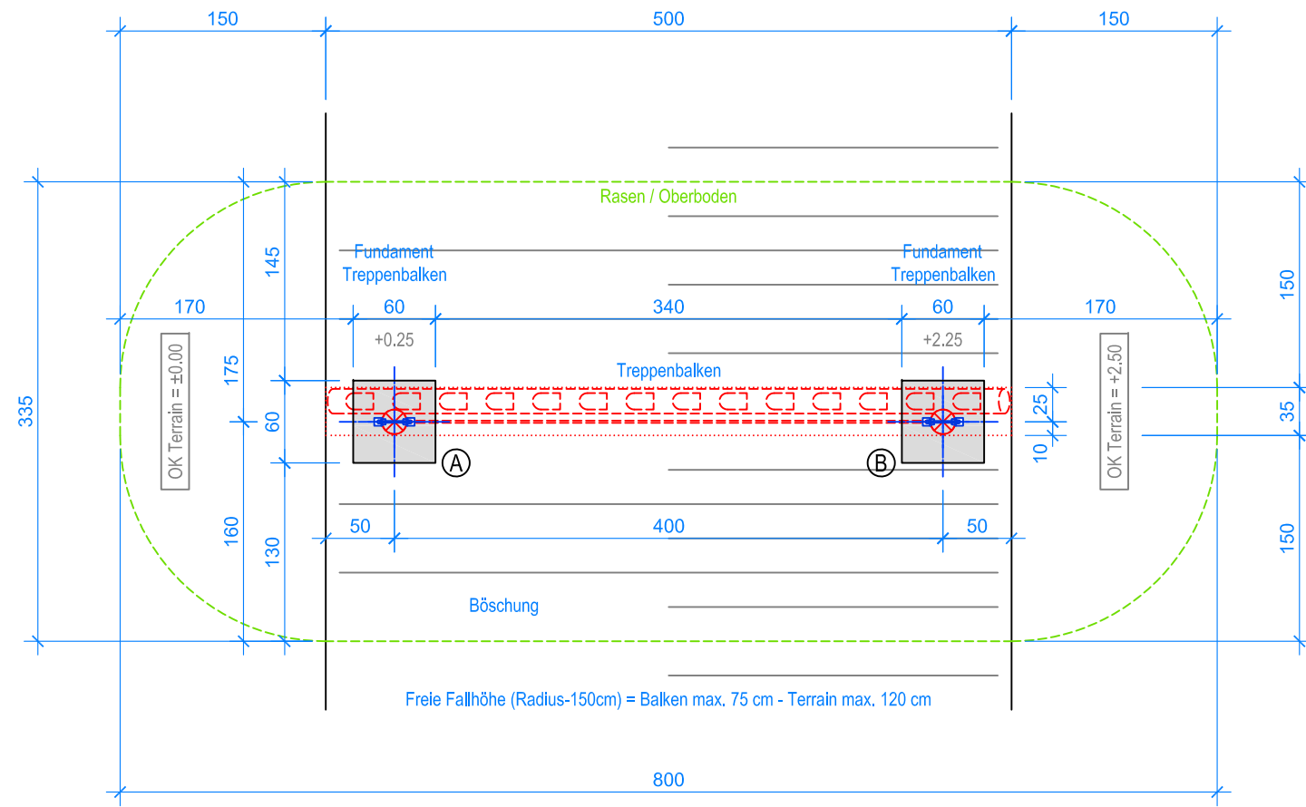
GRUNDRISS 1:50
