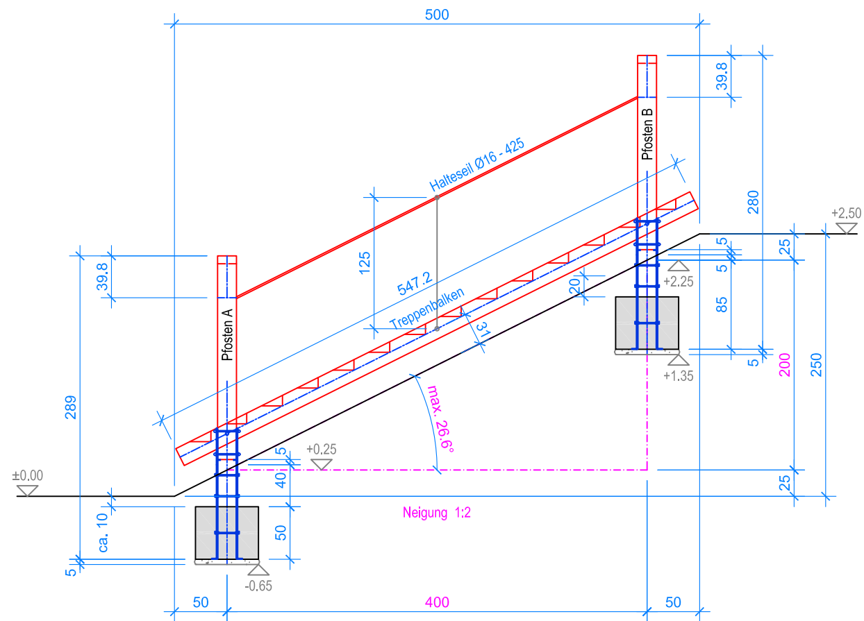
SCHNITT 1:50
