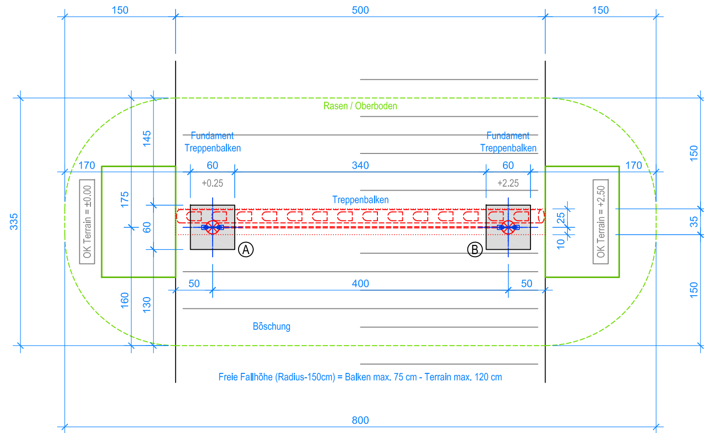
GRUNDRISS 1:50
