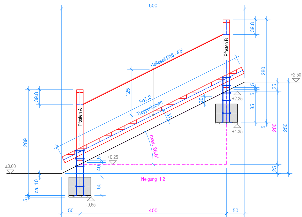
SCHNITT 1:50
