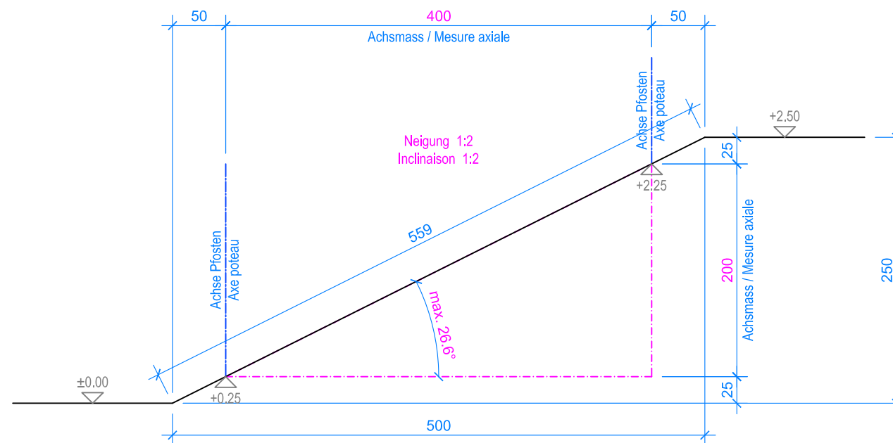
SCHNITT / COUPÉ 1:50
