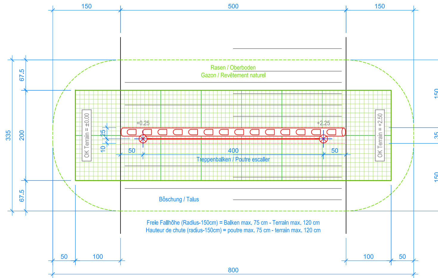
GRUNDRISS / PLAN 1:50
