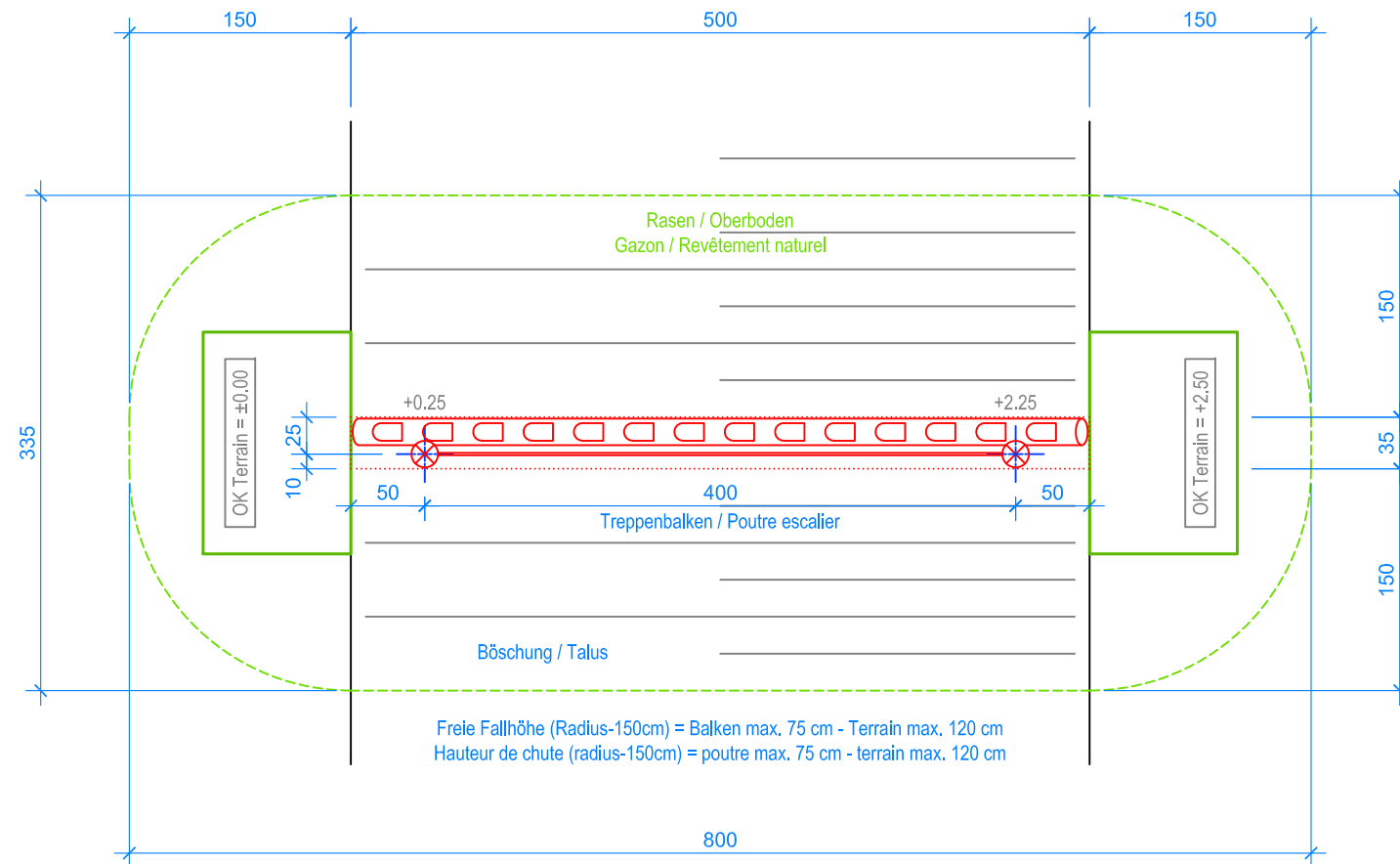
GRUNDRISS / PLAN 1:50
