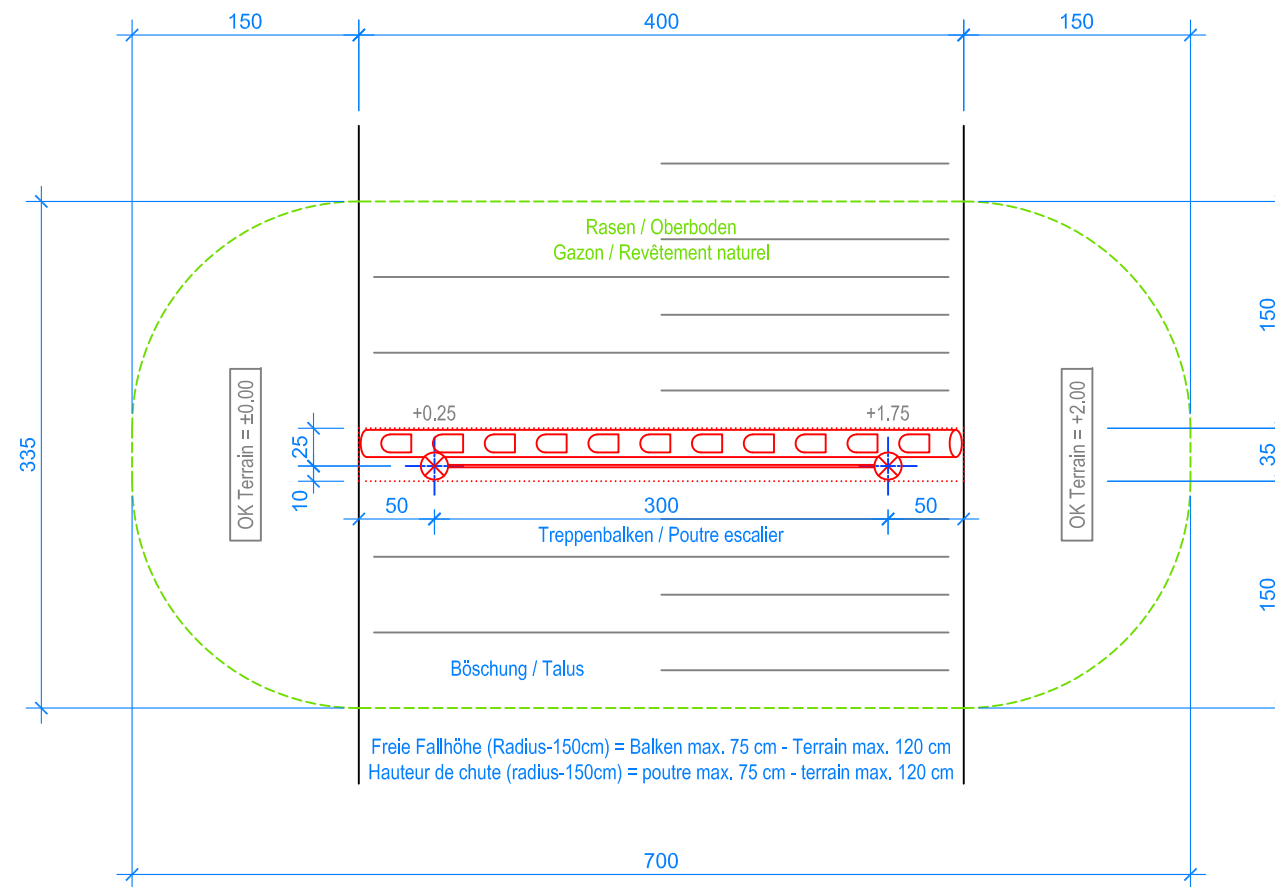
GRUNDRISS / PLAN 1:50
