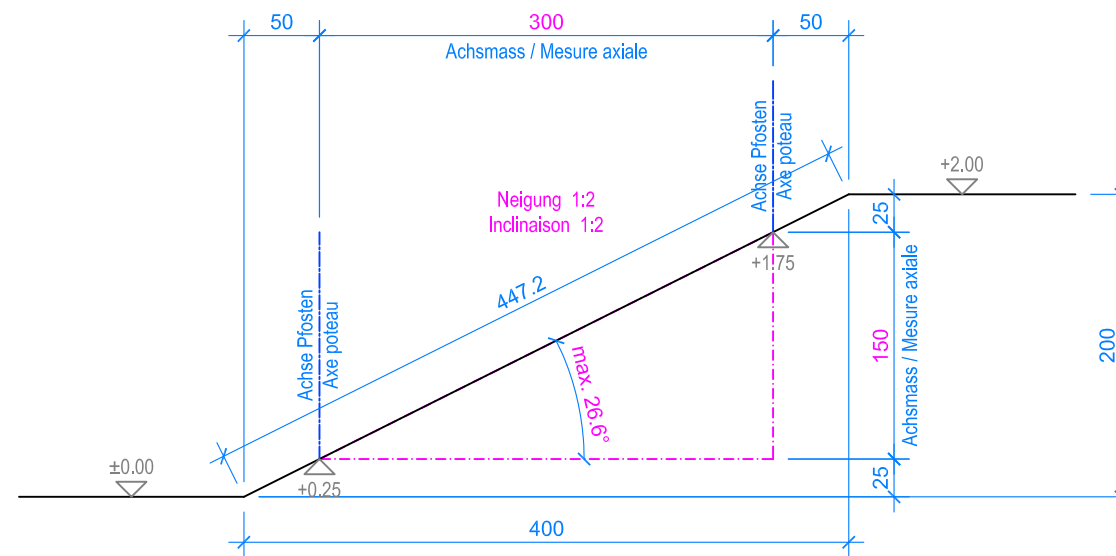
SCHNITT / COUPÉ 1:50
