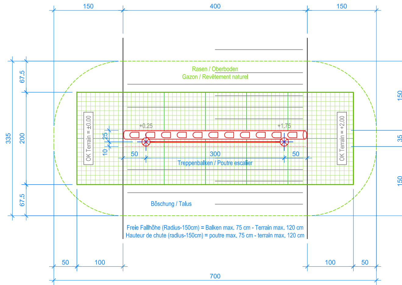
GRUNDRISS / PLAN 1:50
