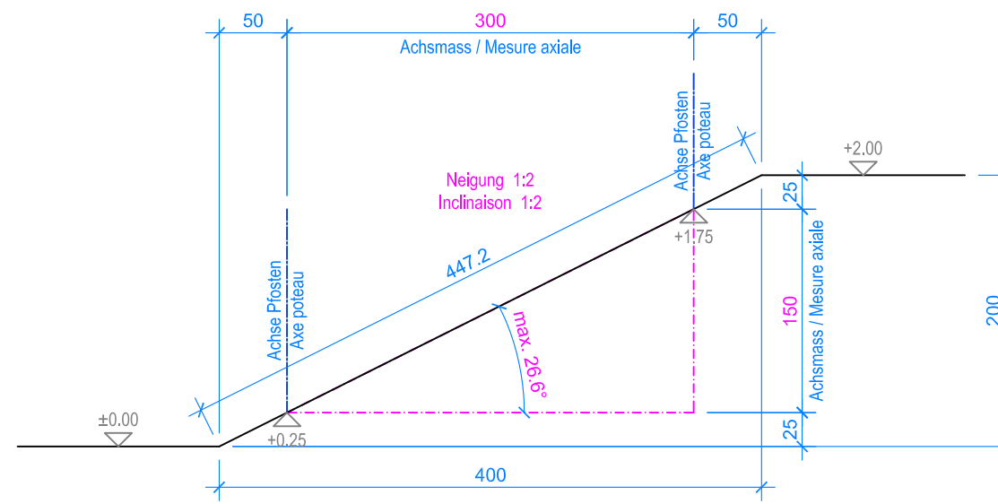
SCHNITT / COUPÉ 1:50
