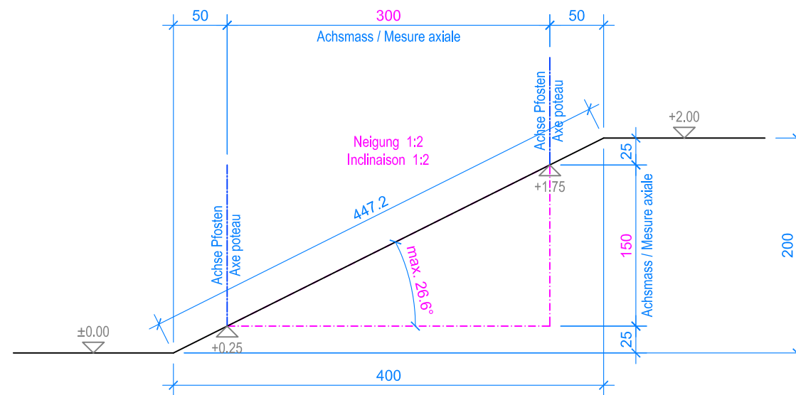
SCHNITT / COUPÉ 1:50
