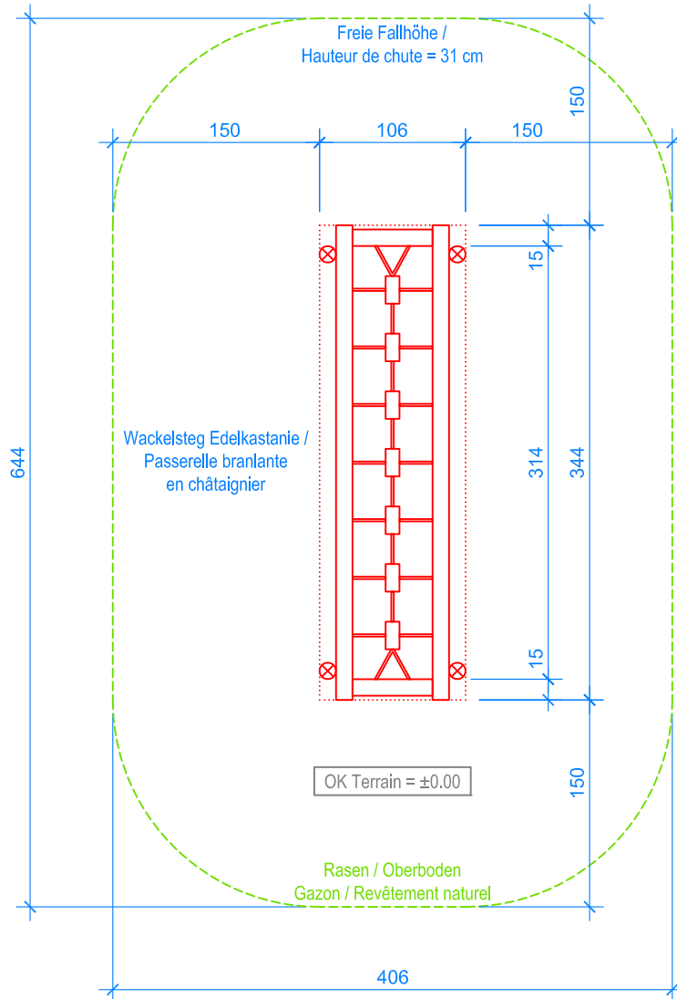
GRUNDRISS / PLAN 1:50
