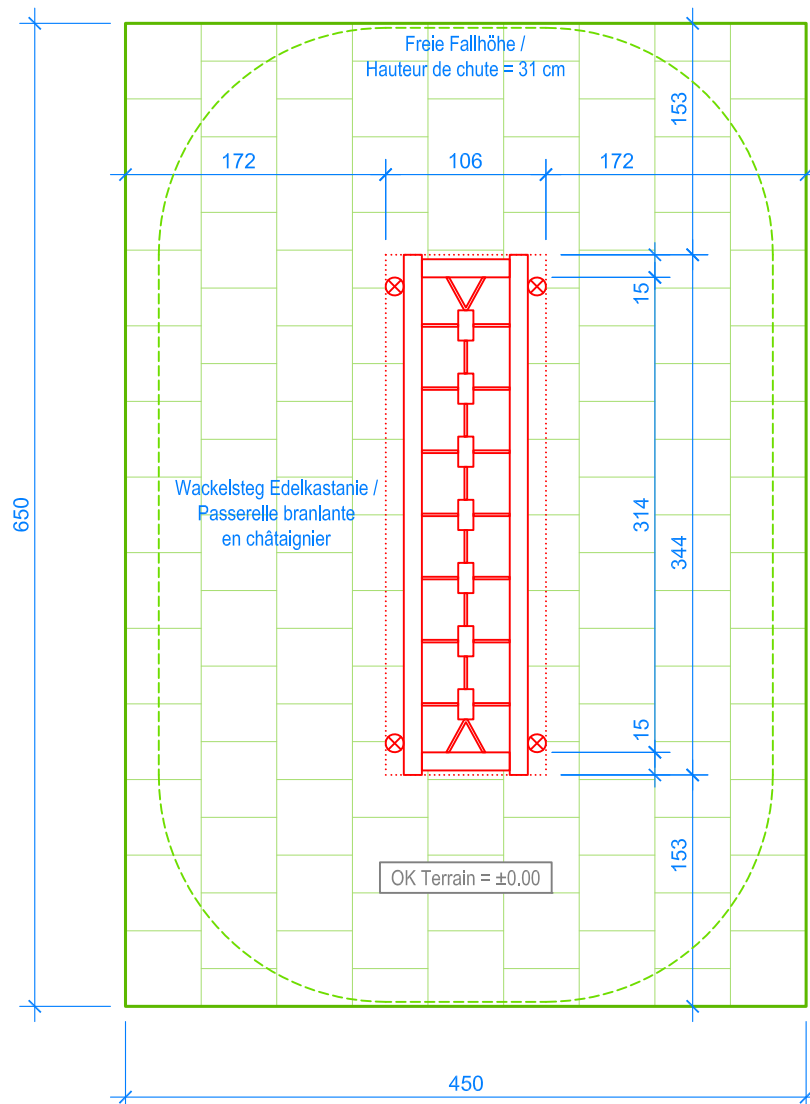
GRUNDRISS / PLAN 1:50
