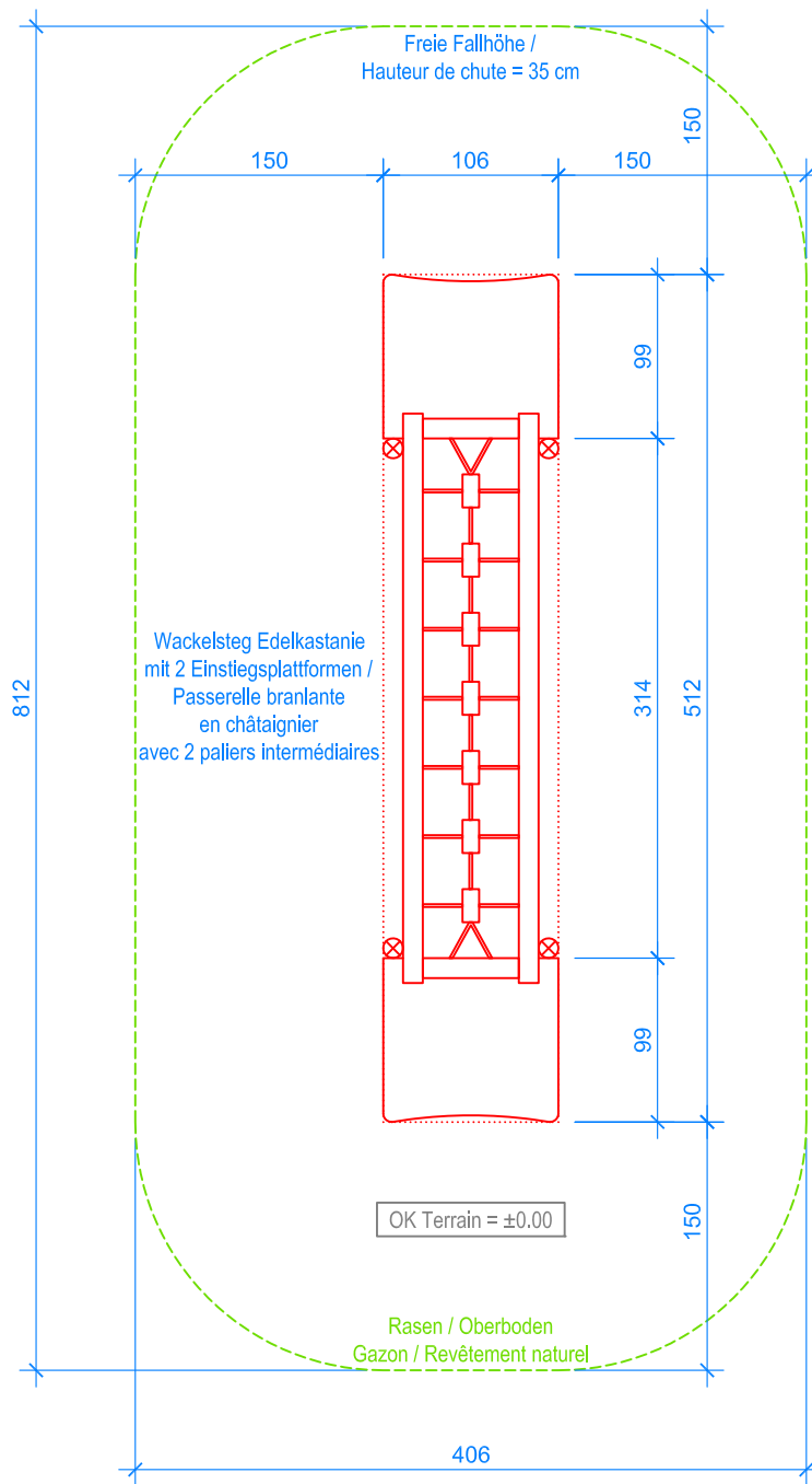
GRUNDRISS / PLAN 1:50
