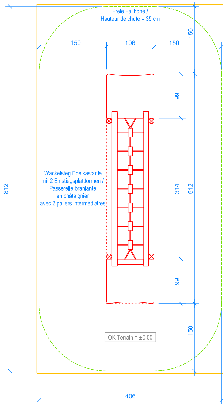
GRUNDRISS / PLAN 1:50
