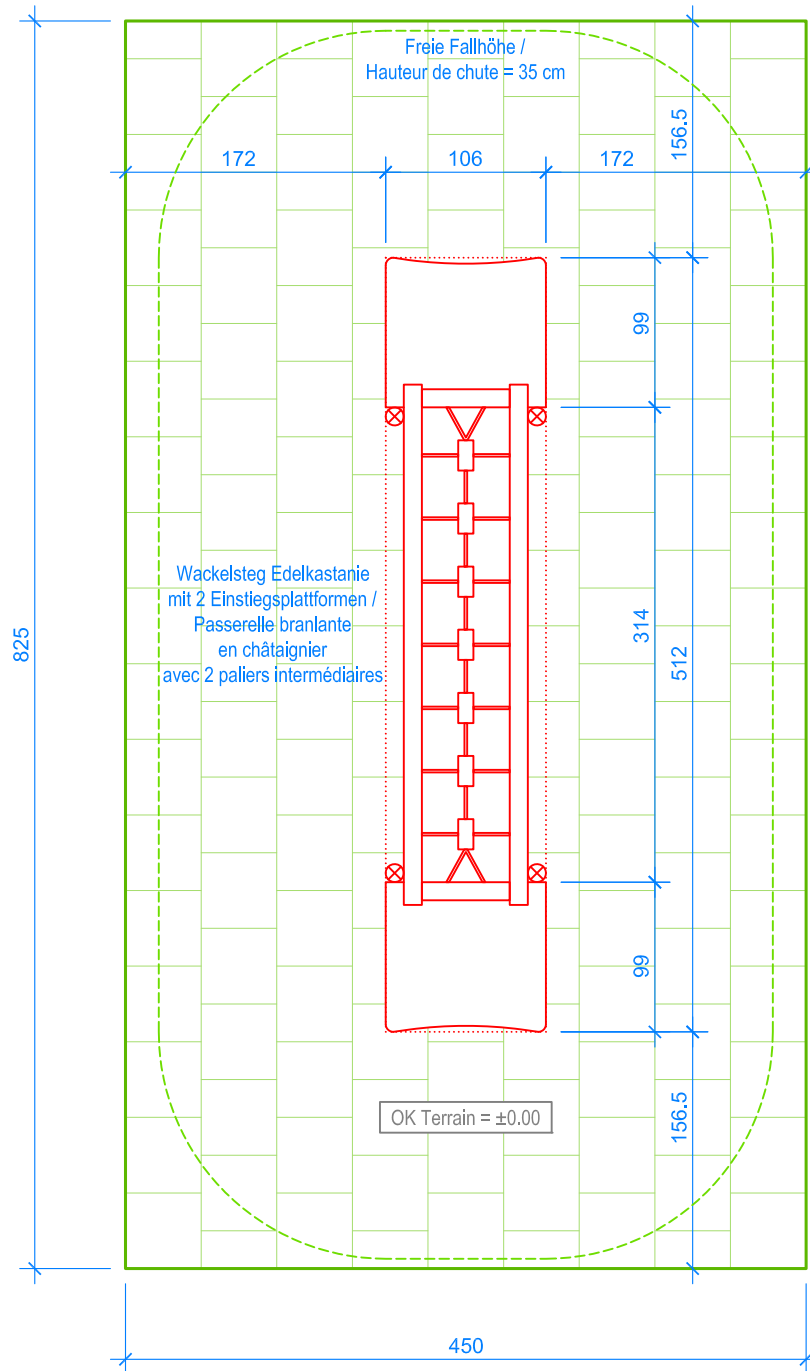
GRUNDRISS / PLAN 1:50
