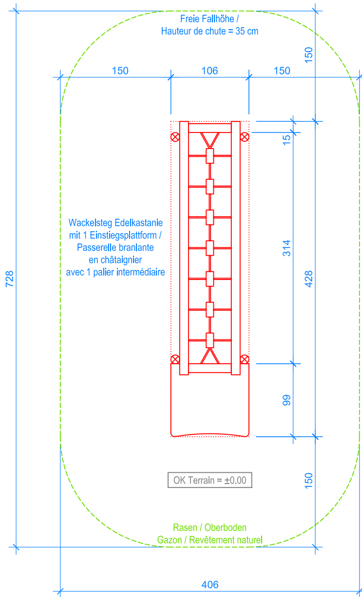
GRUNDRISS / PLAN 1:50
