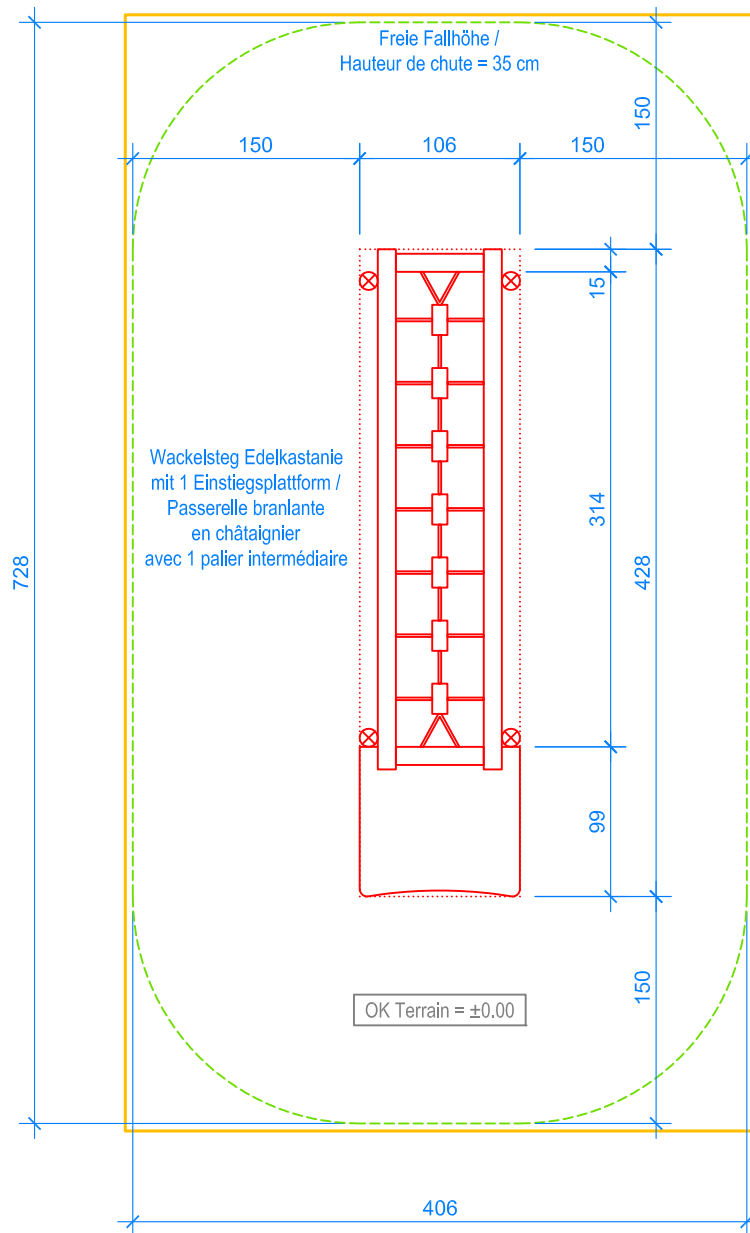
GRUNDRISS / PLAN 1:50
