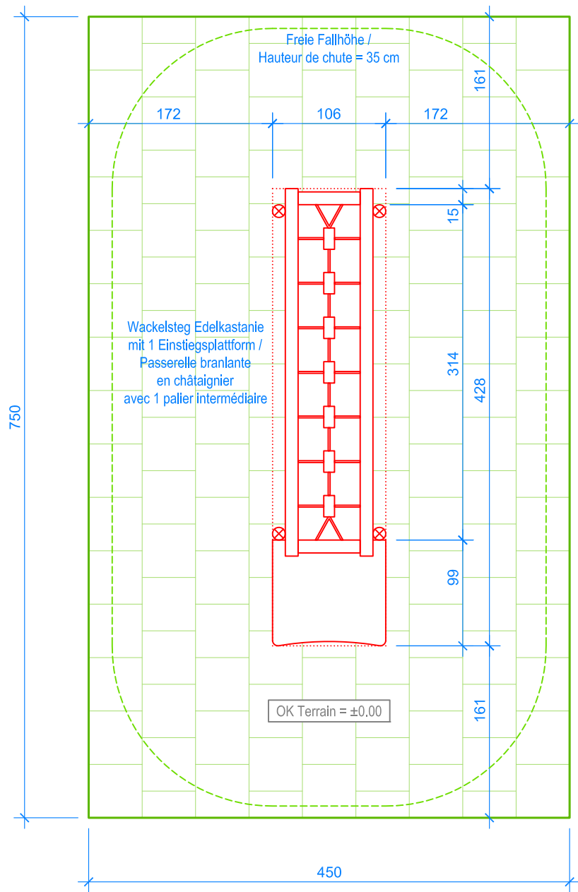
GRUNDRISS / PLAN 1:50
