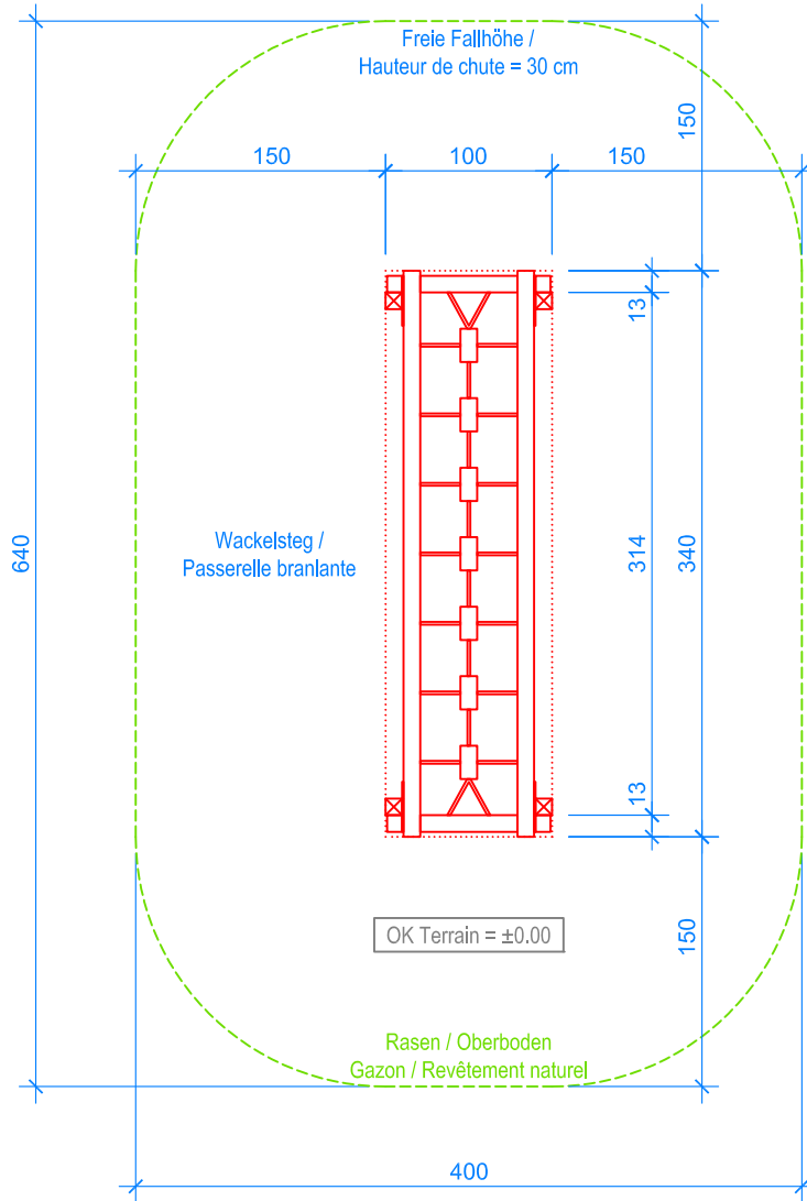
GRUNDRISS / PLAN 1:50
