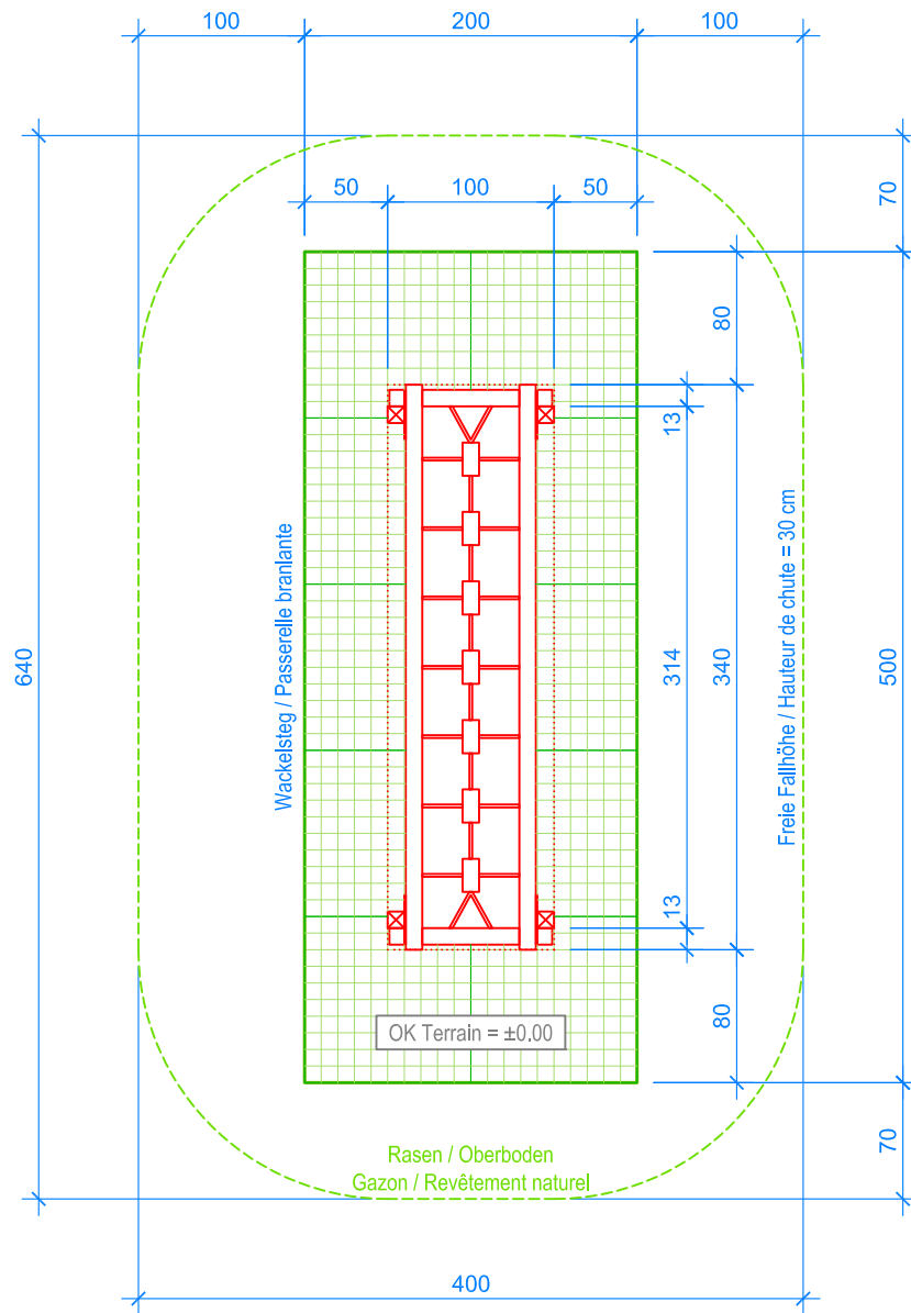
GRUNDRISS / PLAN 1:50
