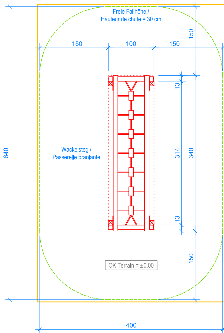
GRUNDRISS / PLAN 1:50
