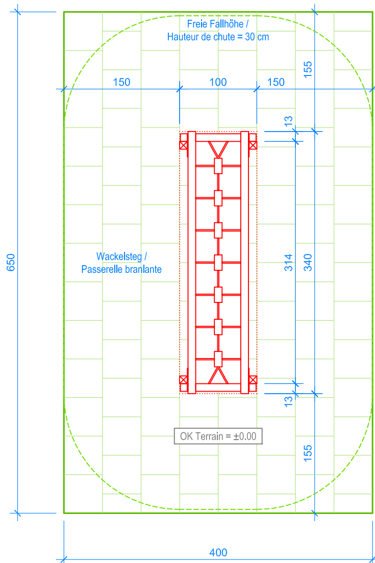
GRUNDRISS / PLAN 1:50
