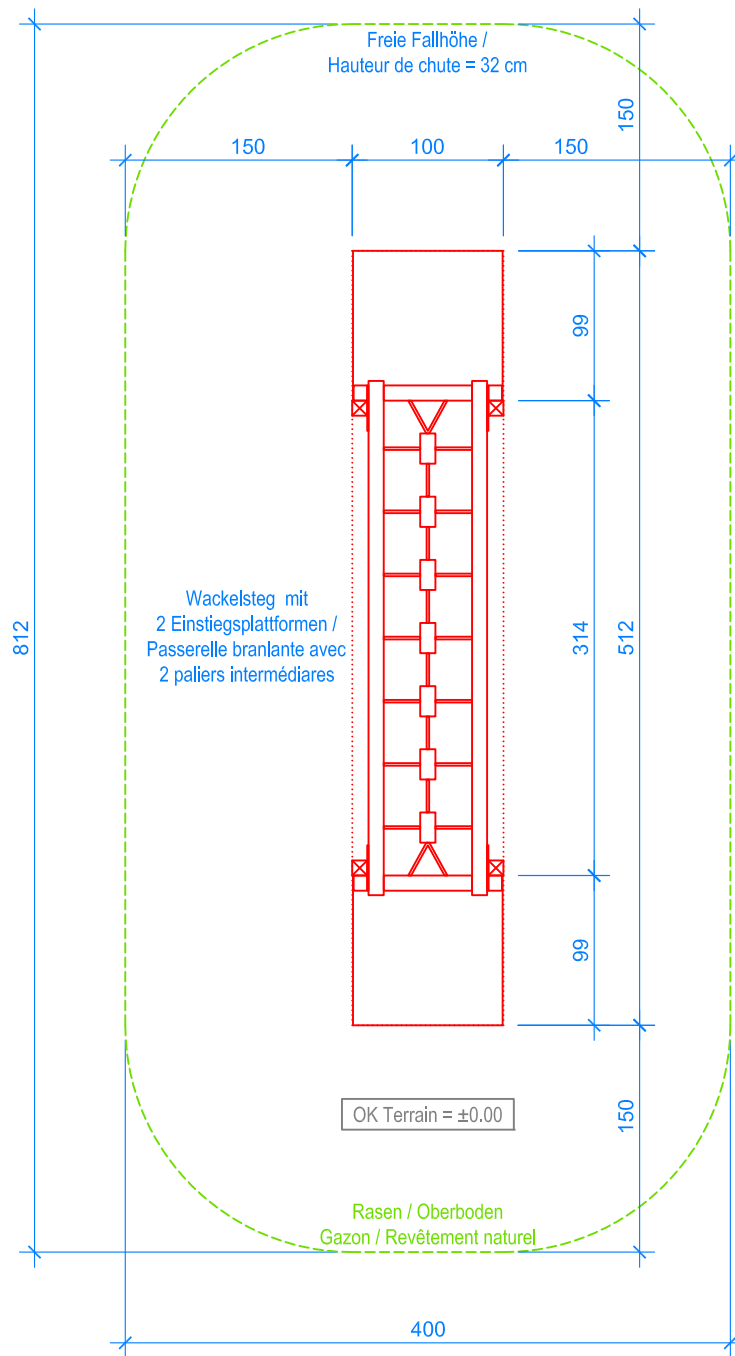
GRUNDRISS / PLAN 1:50
