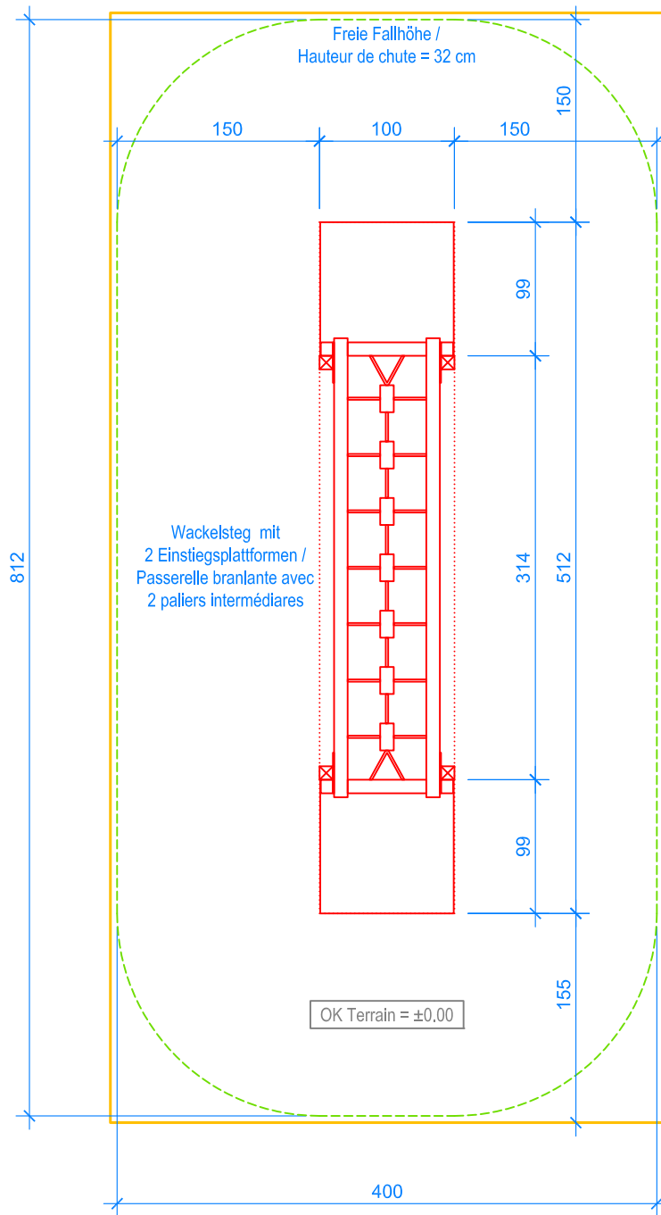
GRUNDRISS / PLAN 1:50
