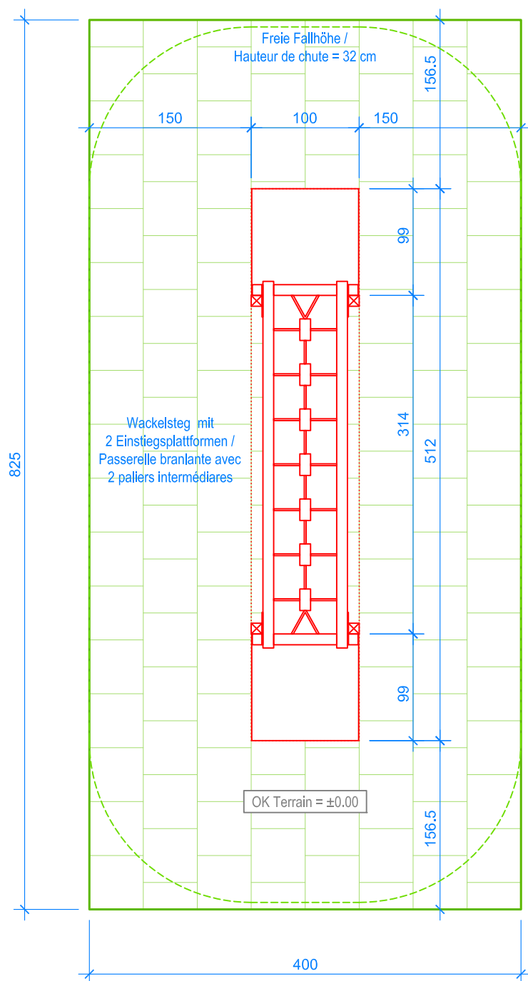
GRUNDRISS / PLAN 1:50
