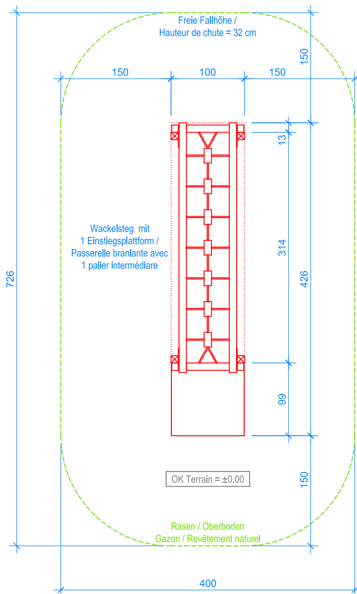
GRUNDRISS / PLAN 1:50
