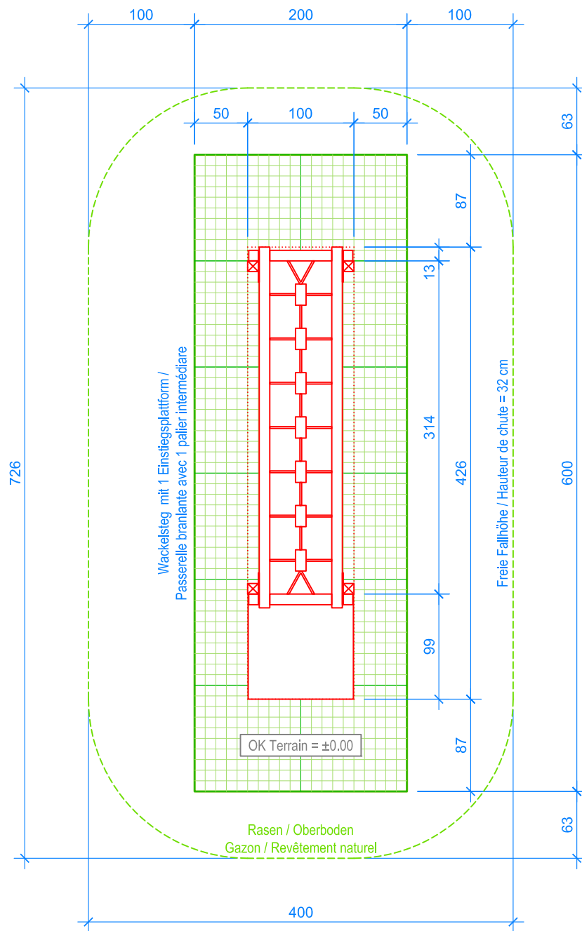
GRUNDRISS / PLAN 1:50
