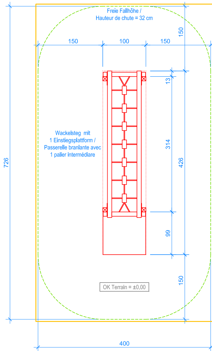
GRUNDRISS / PLAN 1:50
