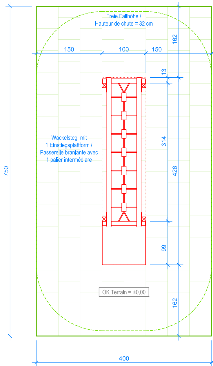
GRUNDRISS / PLAN 1:50
