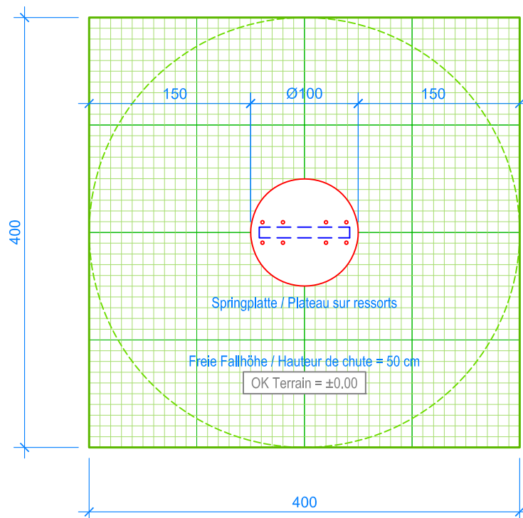
GRUNDRISS / PLAN 1:50
