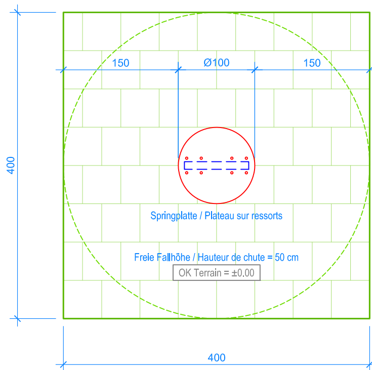
GRUNDRISS / PLAN 1:50
