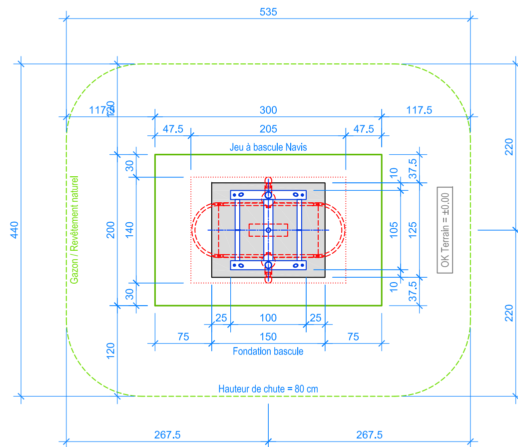
PLAN 1:50
