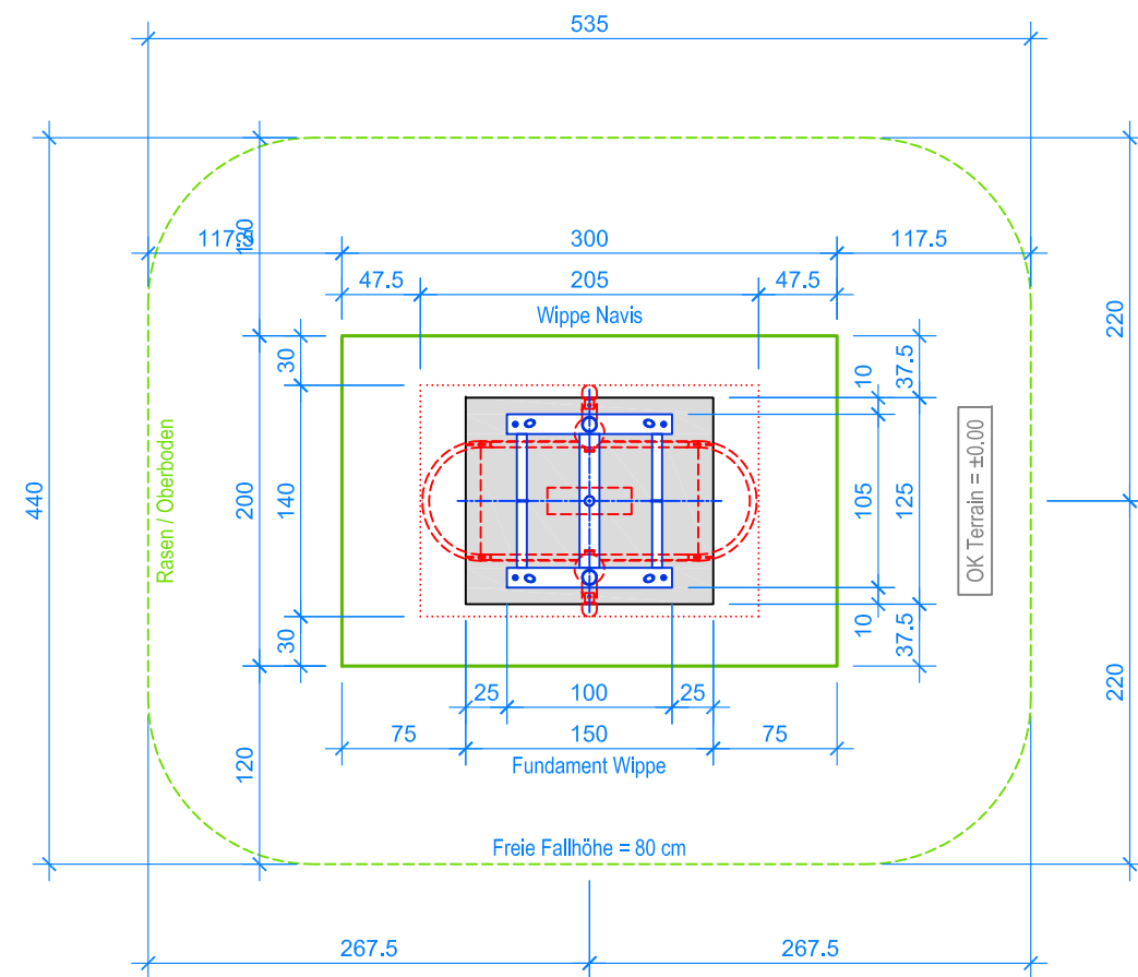
GRUNDRISS 1:50
