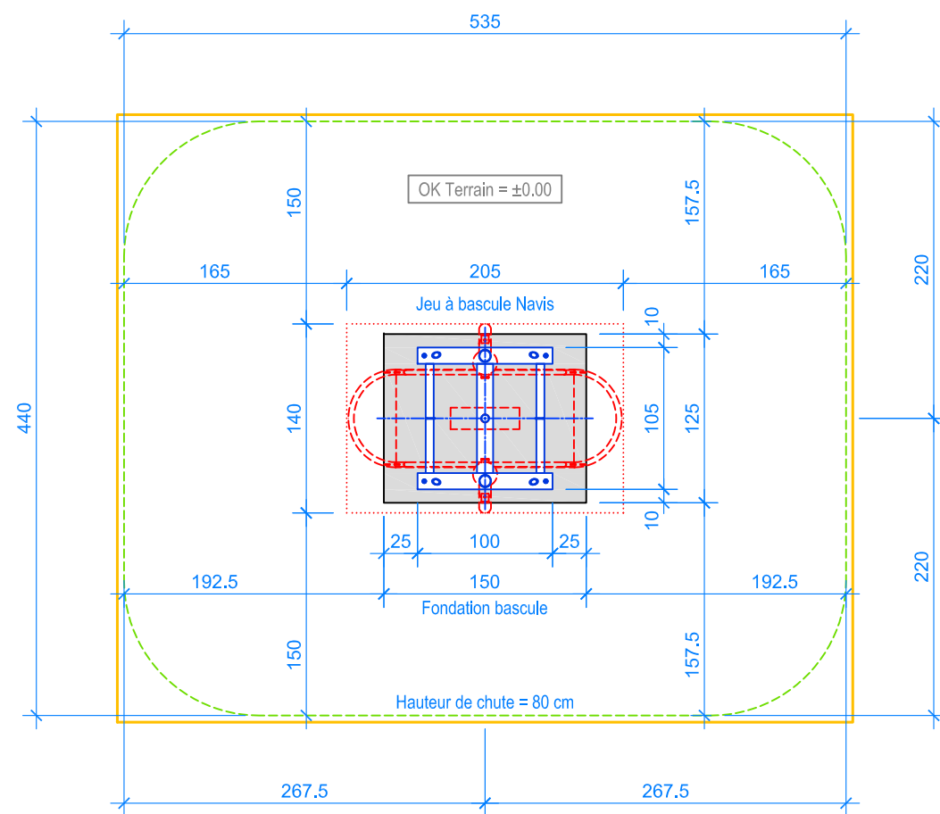
PLAN 1:50
