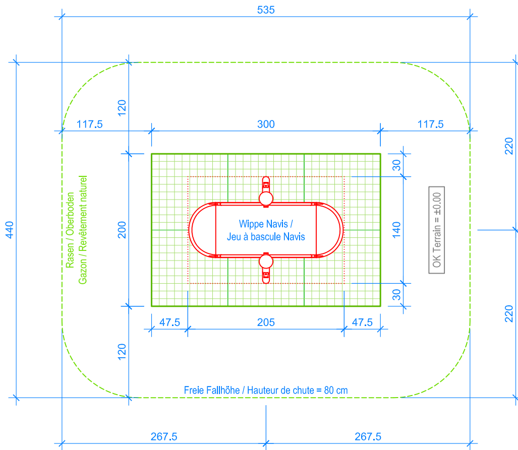
GRUNDRISS / PLAN 1:50
