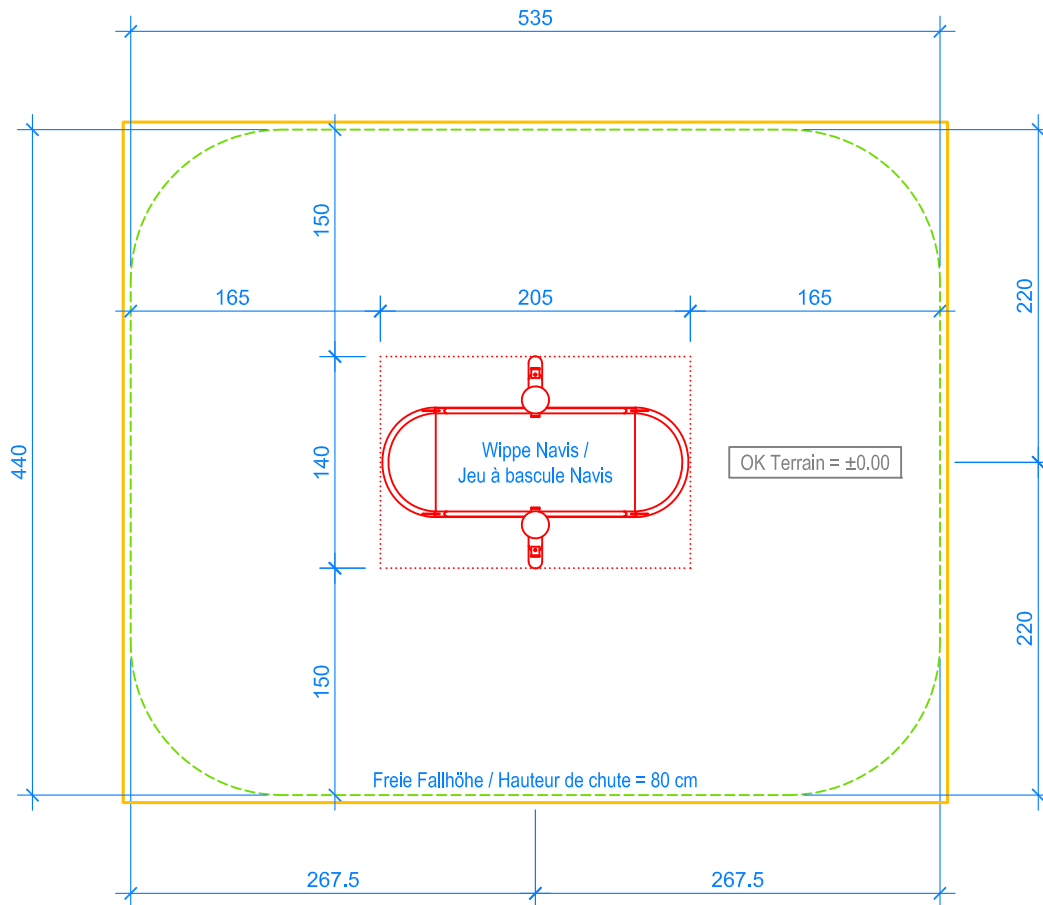
GRUNDRISS / PLAN 1:50
