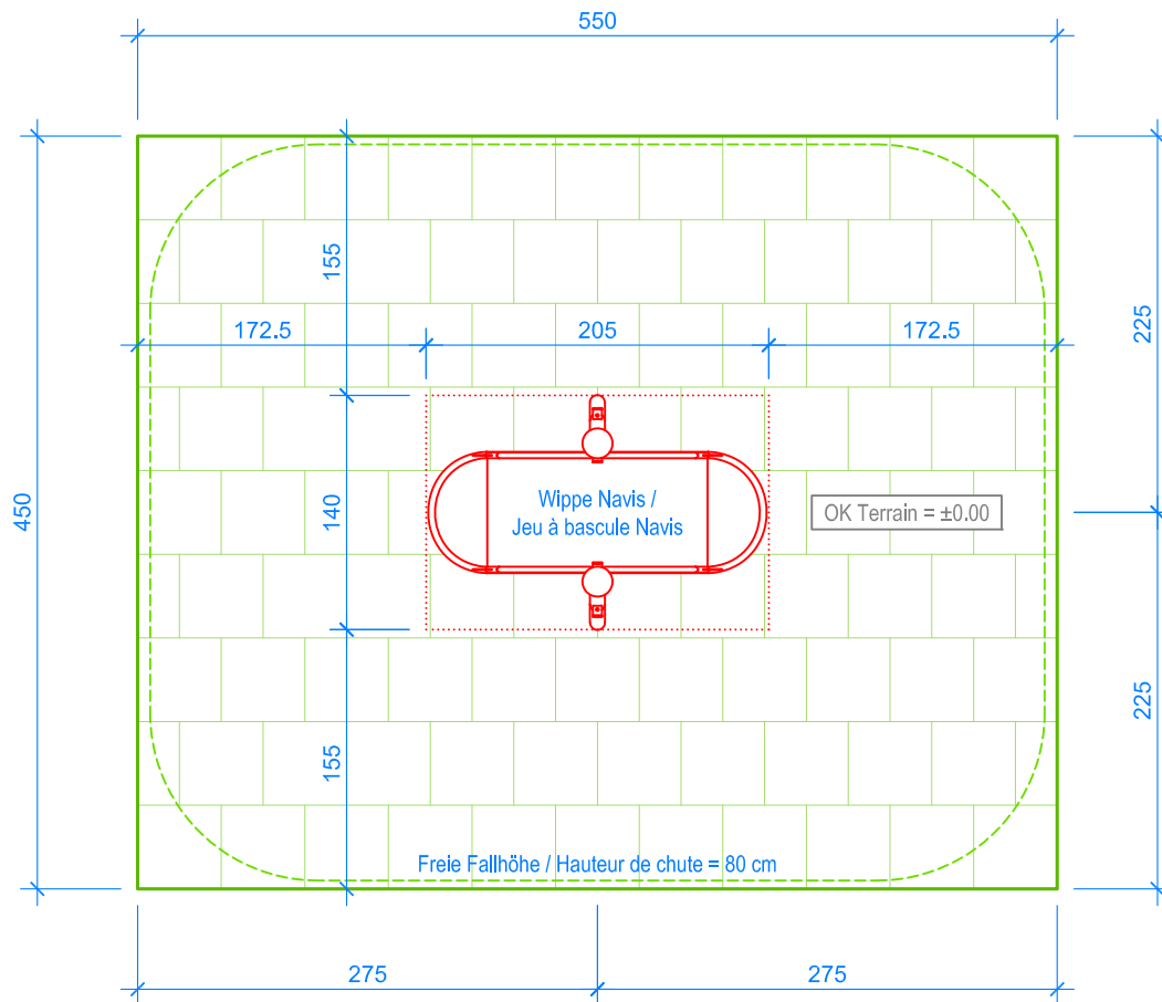
GRUNDRISS / PLAN 1:50
