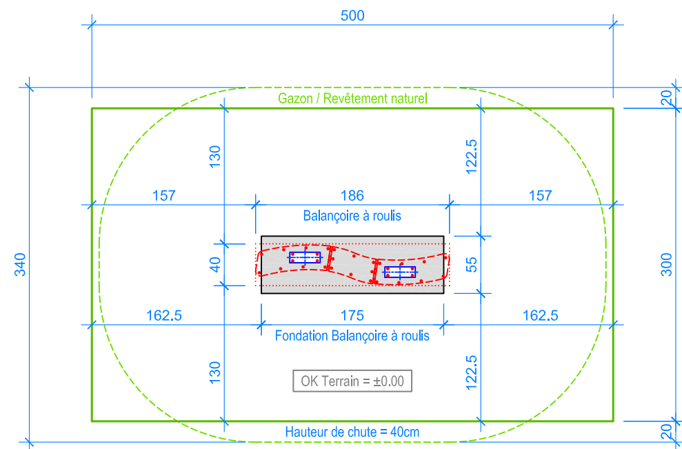
PLAN 1:50
